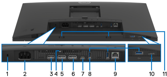
Вид монитора сзади и снизу без стойки
